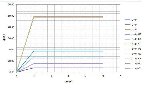
Gambar 11 Kurva Karakteristik Transistor NPNBD139
