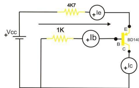
Gambar 13 Rangkaian PNP
