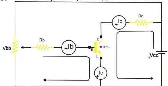
Gambar 10 Rangkaian NPN
