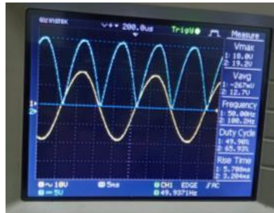
Gbr.13 hasil pengujian penyearah gelombang
