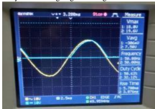
Gbr.12 hasil pengujian penyearah setengah gelombang
