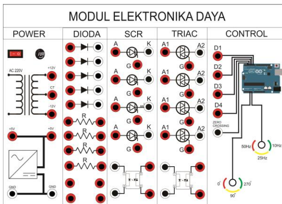
Gbr.8 Perancangan keseluruhan
